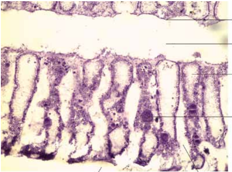
SP2.4. :Coupe de Grantia
