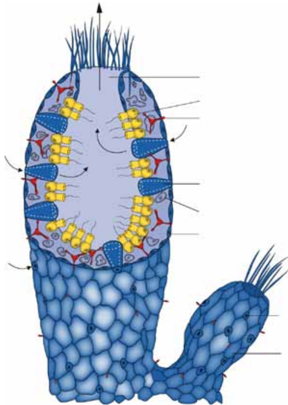
SP 2.1. Aspect général d'un spongiaire
