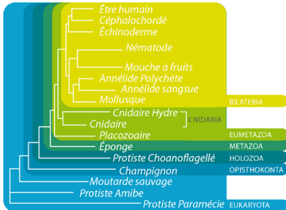
SP. 3.4. Arbre phylogénétique du règne animal, incluant le premier Spongiaire dont le génome complet a été séquencé, Amphimedon queenslandica (d'après Srivastava et al 2010).
