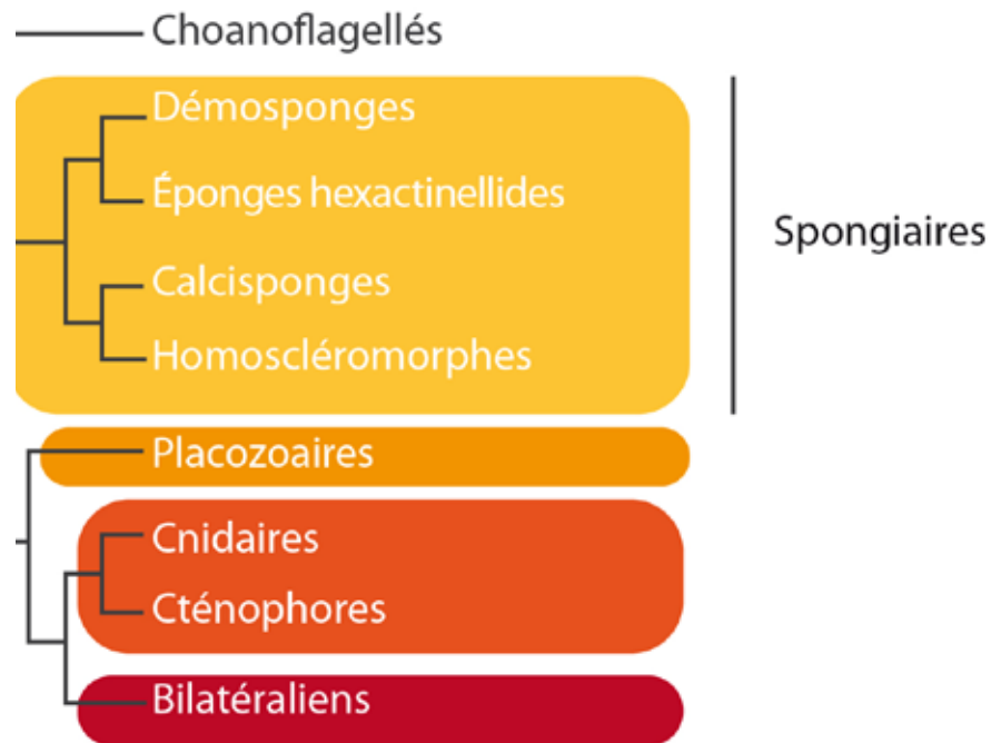
SP.3.3. : Arbre phylogénétique obtenu sur base du séquençage de 129 gènes correspondant à un total de 30257 acides aminés (d'après Telford 2009). Cet arbre montre qu'on distingue 4 groupes d'éponges, et les relations entre ces différents groupes.
