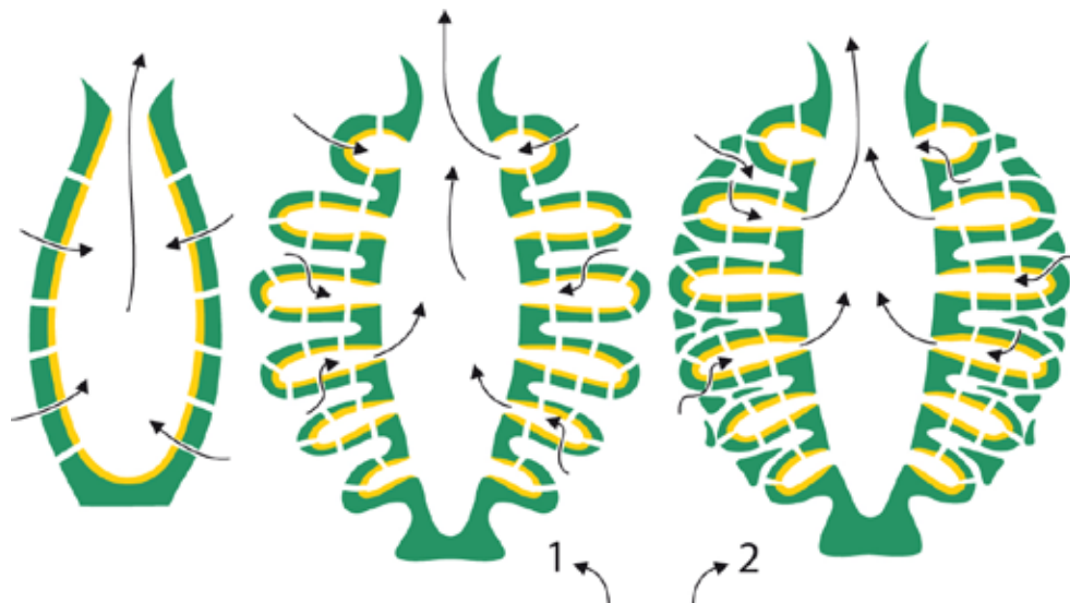
SP 3.1. Variations de structure chez les Eponges ; en jaune, le revêtement interne de choanocytes formant des canaux dans l'animal et permettant ainsi les mouvements d'eau. En vert, le revêtement externe formés de différents types cellulaires et de mésoglye. De gauche à droite, on dénomme ces types de structure ascon, sycon et leucon
