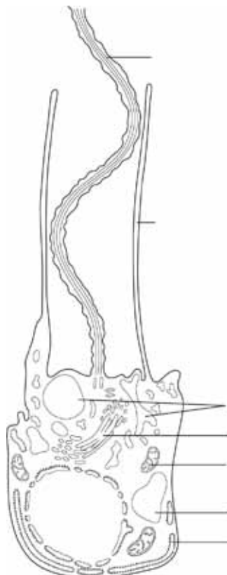
SP 2.3. Structure d'un choanocyte
