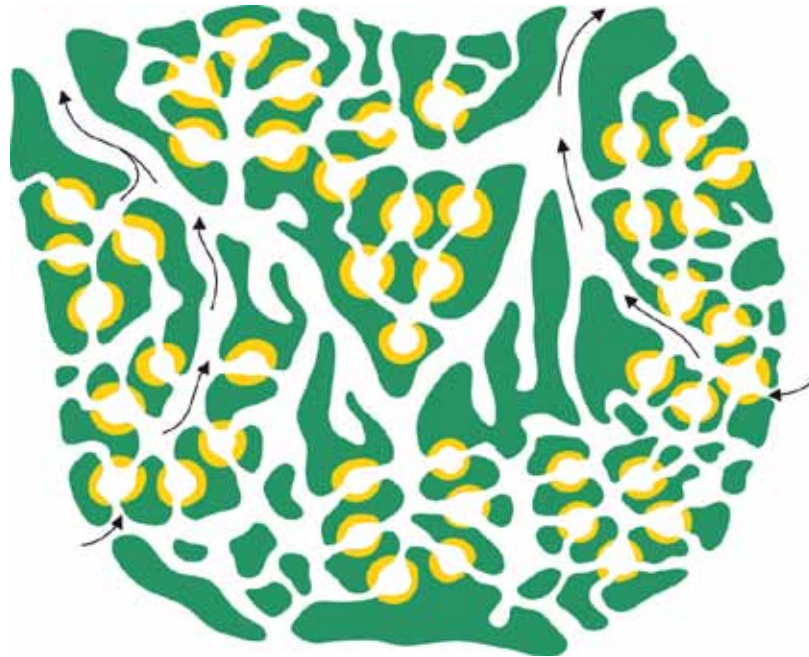
SP 3.2. Spongiaire type leucon; en jaune, les chambres à choanocytes
