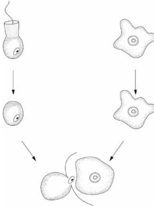
SP 2.5. Reproduction sexuée chez les spongiaires
